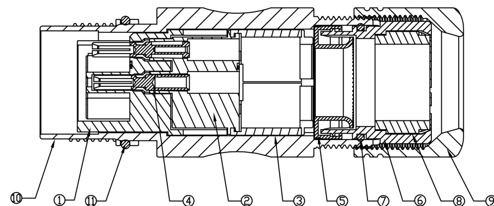
截面A-A 2:1
