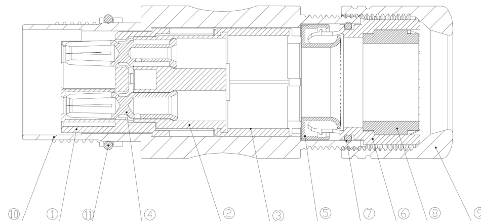
截面A-A 2:1
