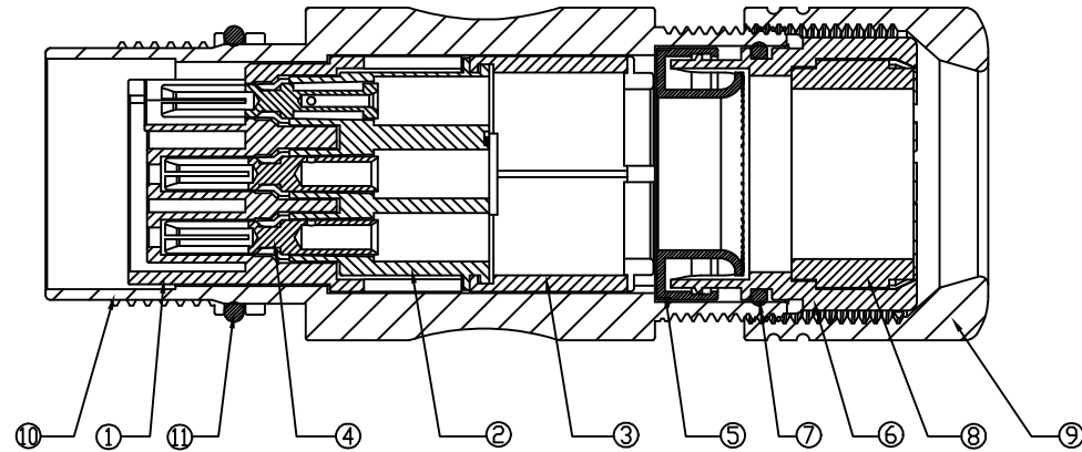
截面A-A 2:1
