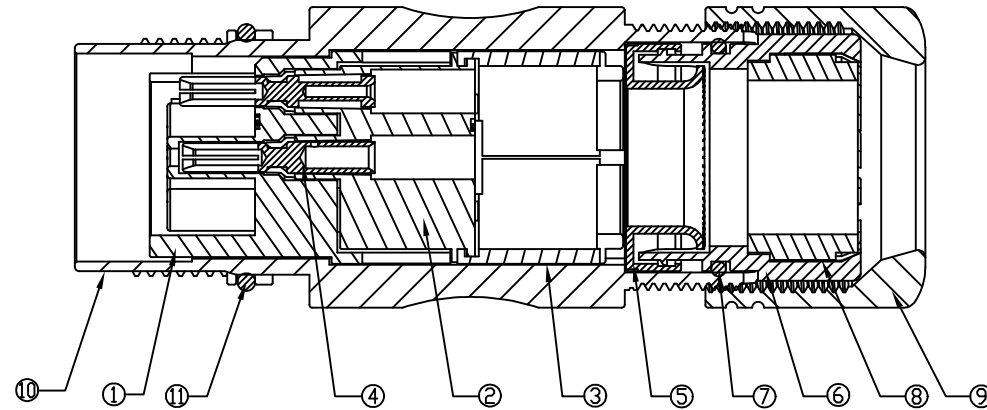
截面A-A 2:1
