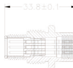
端子铆压高度
